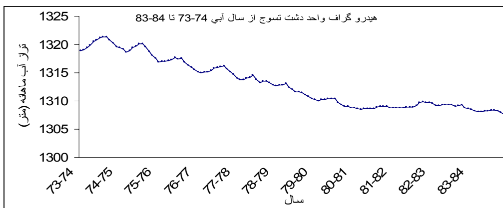
شکل ۴- هیدروگراف واحد آب زیرزمینی دشت تسوج از سال آبی ۷۴-۷۳ تا ۸۴-۸۳
